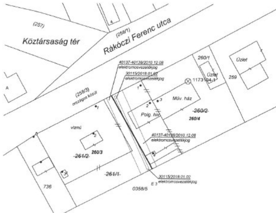
változási vázrajz, tervezett telekhatár rendezés
