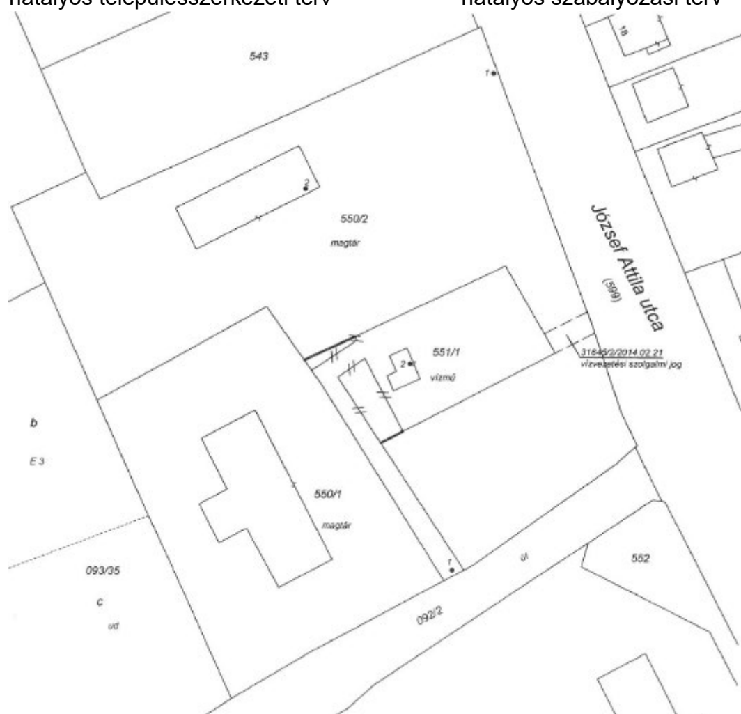
változási vázrajz, tervezett telekhatár rendezés
