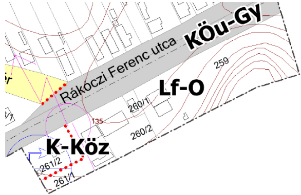
hatályos szabályozási terv
