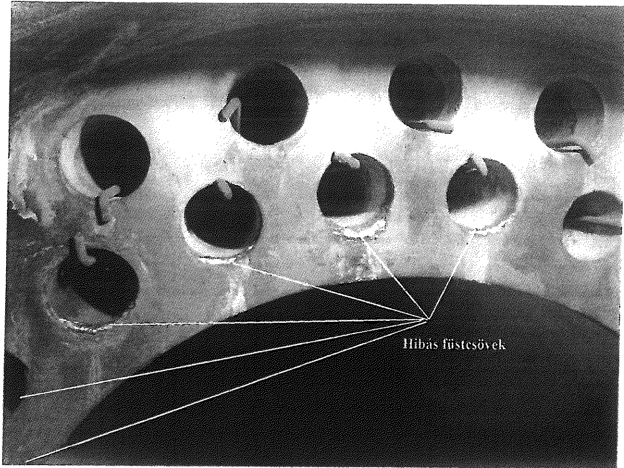
Folyás, szivárgó füstcsövek a belső körön és bal oldali területen
