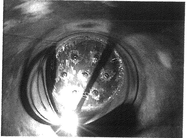
I. számú kazán – lángcső fenéklemez hátul új behegesztett támasztó rudakkal - Nyomáspróba jkv. szerint
