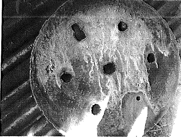
I. számú kazán – kivágott lángcső fenéklemez,
